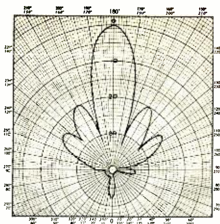
Fig. 3. H-plane pattern for 6' antenna.
