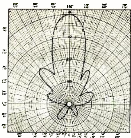
Fig. 2. E-plane pattern for 6' antenna.
